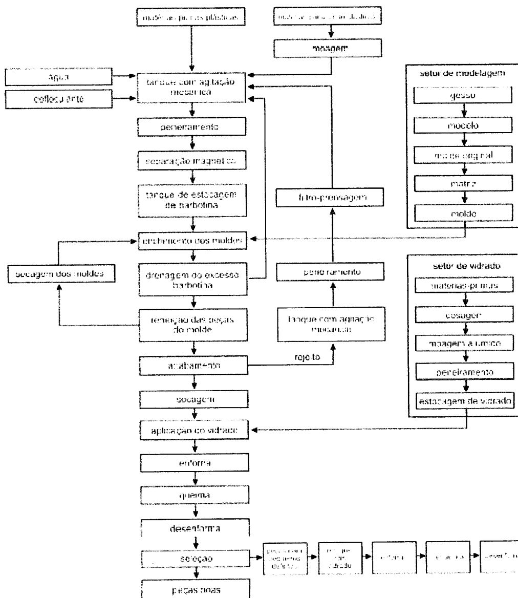
FLUXOGRAMA 2 - PROCESSO DE FABRICAÇÃO DE SANITÁRIOS
