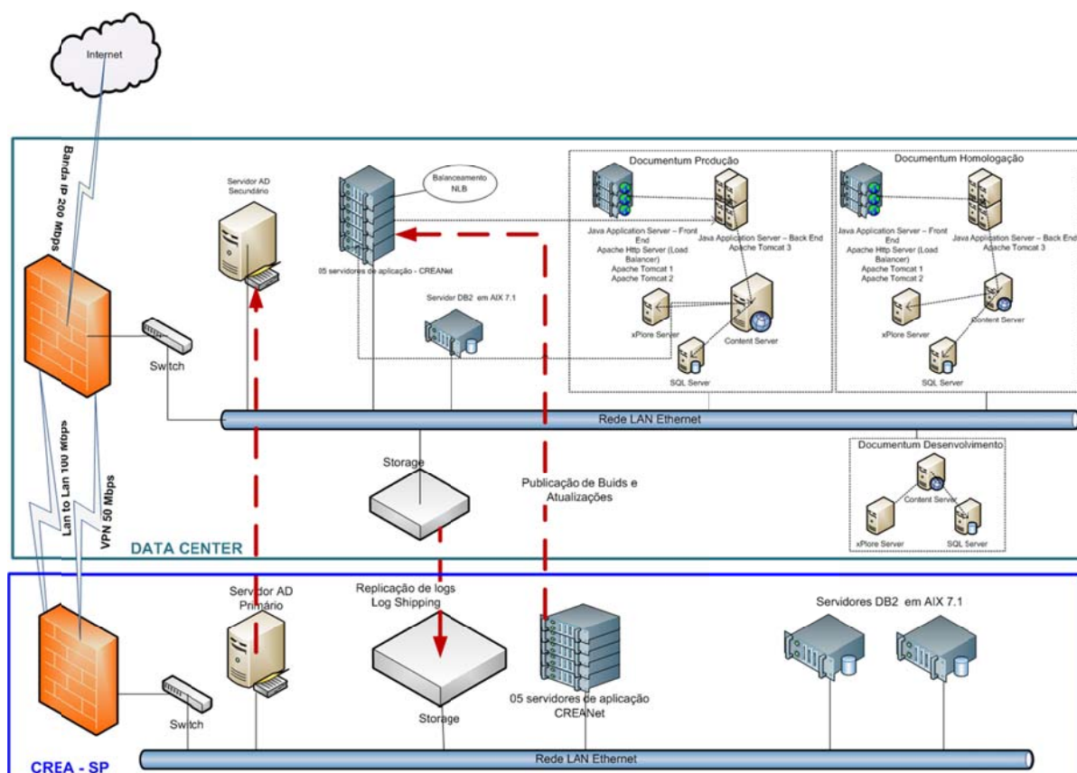
FIGURA 25. ARQUITETURA DATA CENTER
